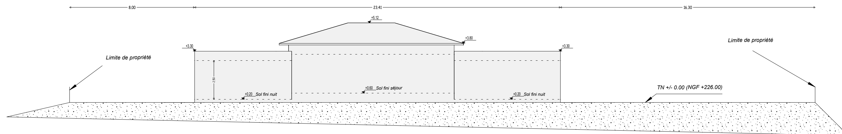
Plan en coupe de la construction et du terrain Echelle 1/150° PC 03
