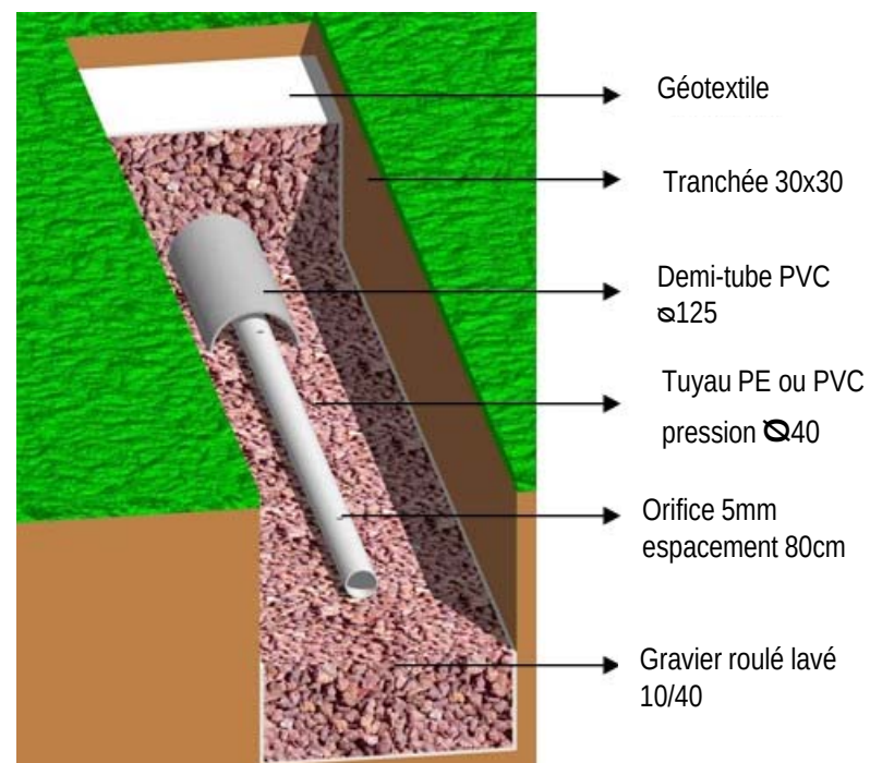
Schéma de coupe de la tranchée
