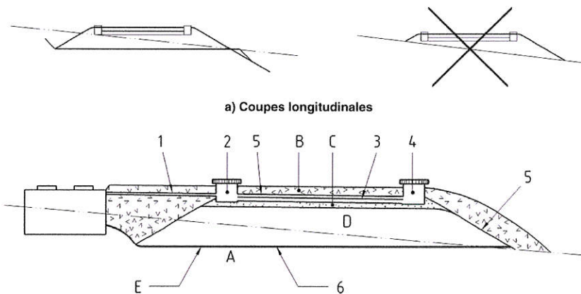
Figure 9 — Exemple de tertre d'infiltration hors sol
